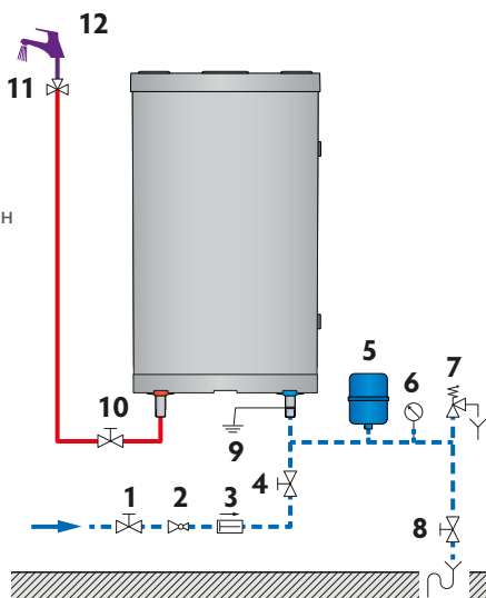
Вертикальный монтаж
